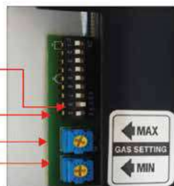
Рисунок 15. DIP-переключатели
