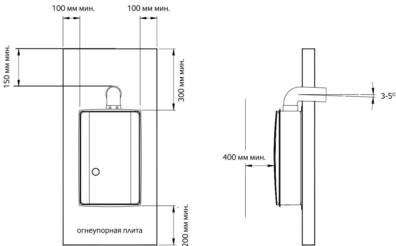
Рисунок 11. Установка котла
