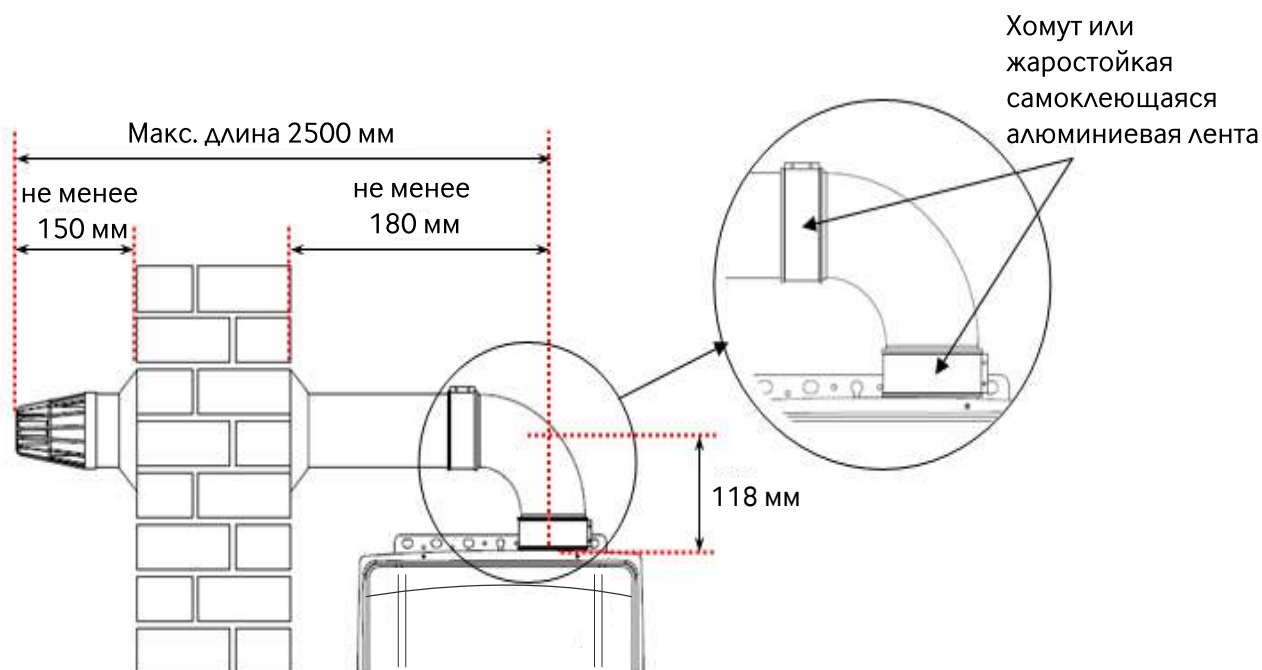
Рисунок 12. Установка дымохода
